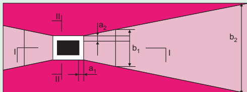
План вертодрома
